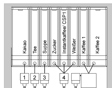
CFS 500 EC/ES Variante 8407 EG EC Variante 8407 EG ES
