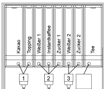
CFS 500 EC/ES/EO Variante 8301 EC Variante 8301 ES Variante 8301 EO
